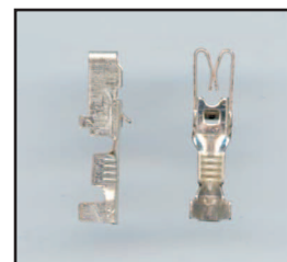
Crimp-Kontakte
