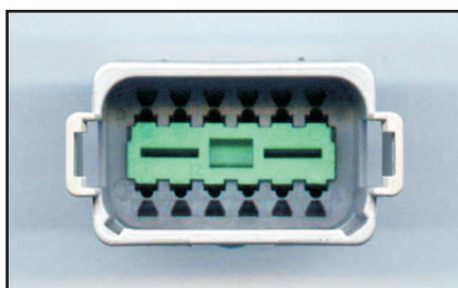
Stiftgehäuse mit Kontaktverriegelung von vorne
