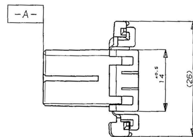
Buchsengehäuse
