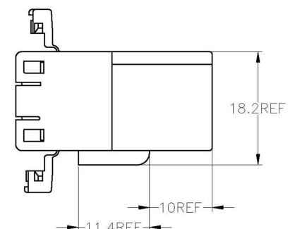
Stiftgehäuse
