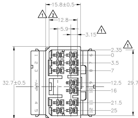
Stiftgehäuse
