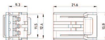
Buchsengehäuse
