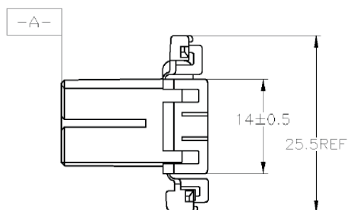
Buchsengehäuse
