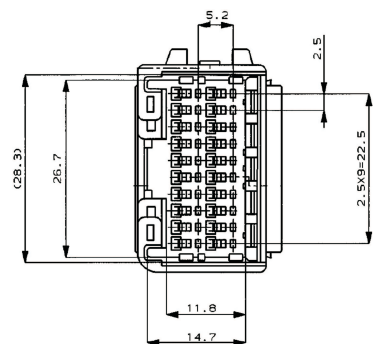
Stiftgehäuse
