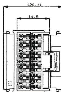
Buchsengehäuse
